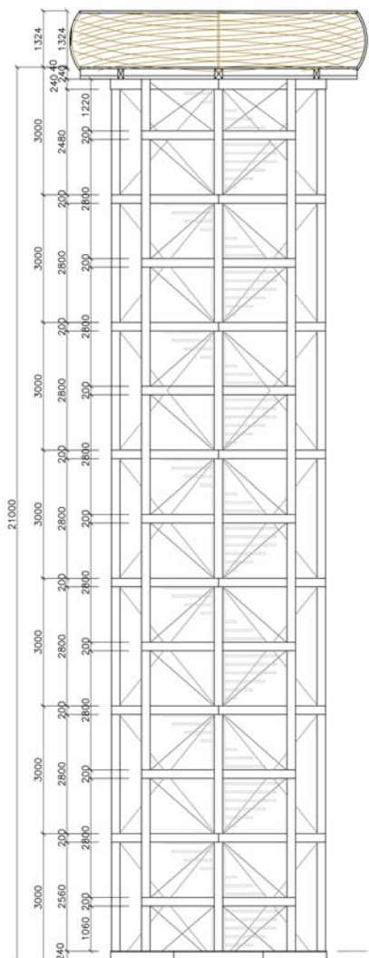
Konstrukční pohled na novou rozhlednu na Světlém vrchu, která bude v rámci projektu "Přeshraniční spolupráce" postavena.
